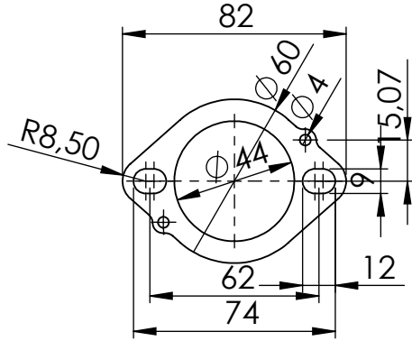
S.s. Flange Cod.204569R
