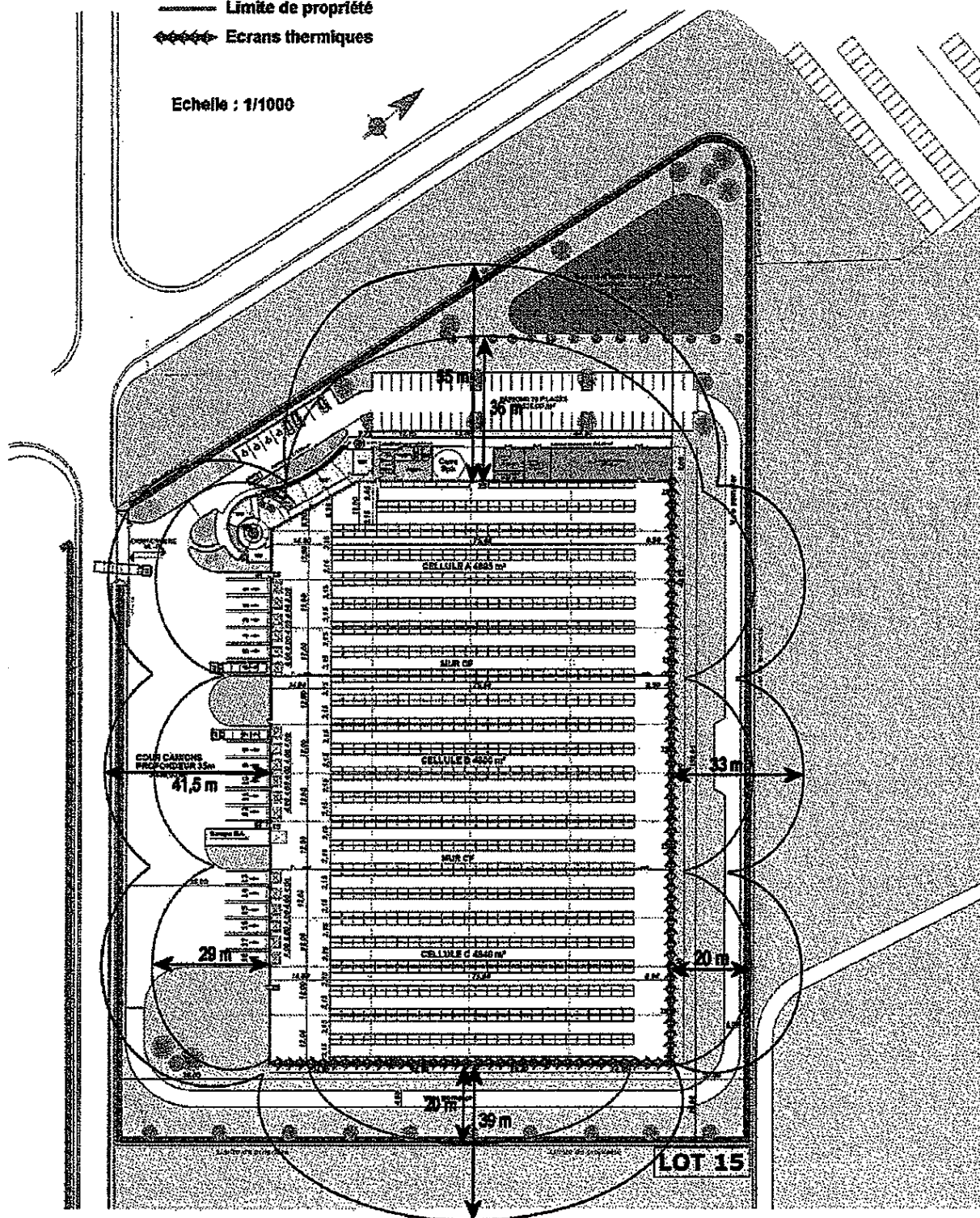
Figure 1 : Plan des flux thermiques
