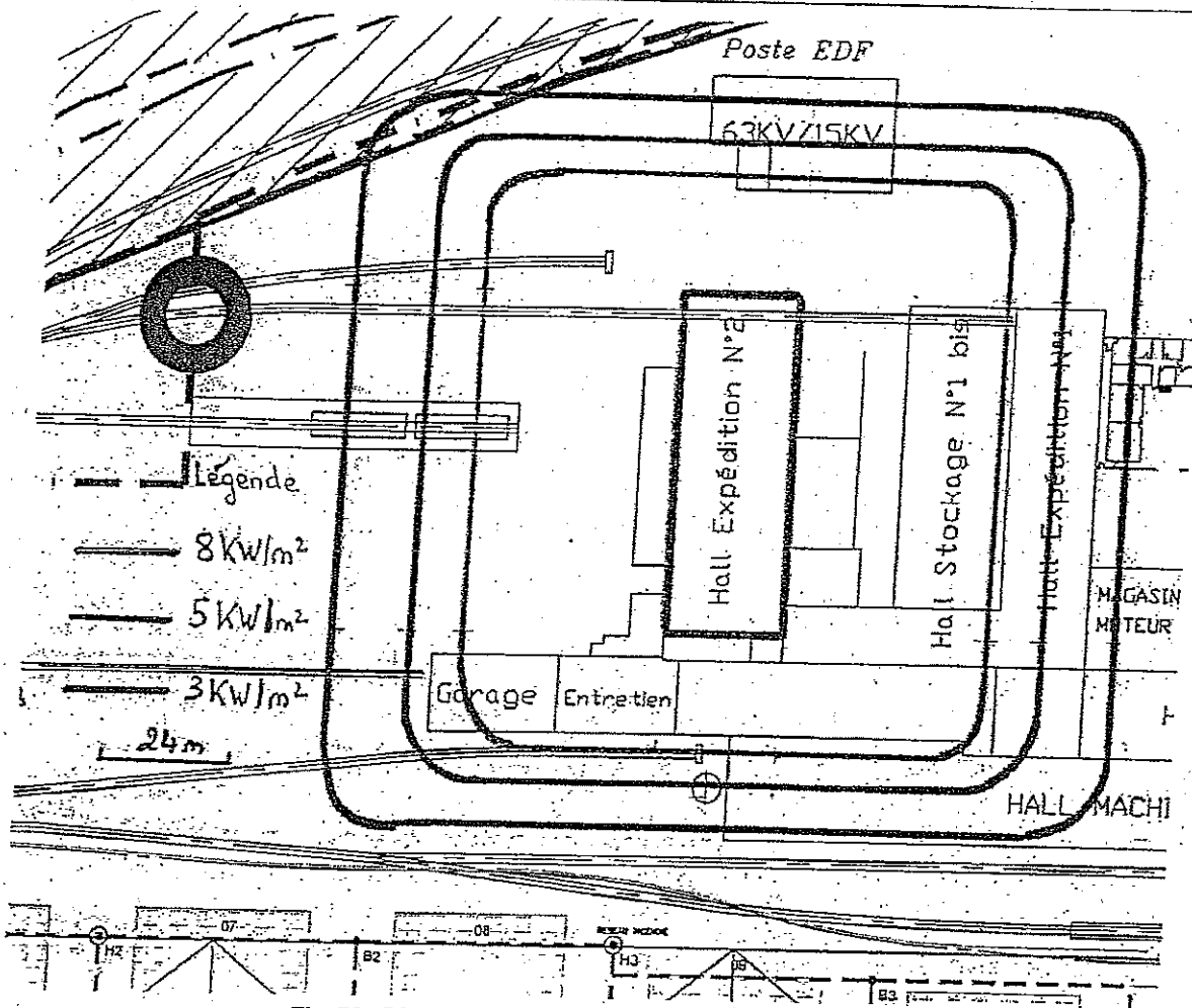
Fig. 72 : Distance d'effets pour l'incendie sur le hall 2
