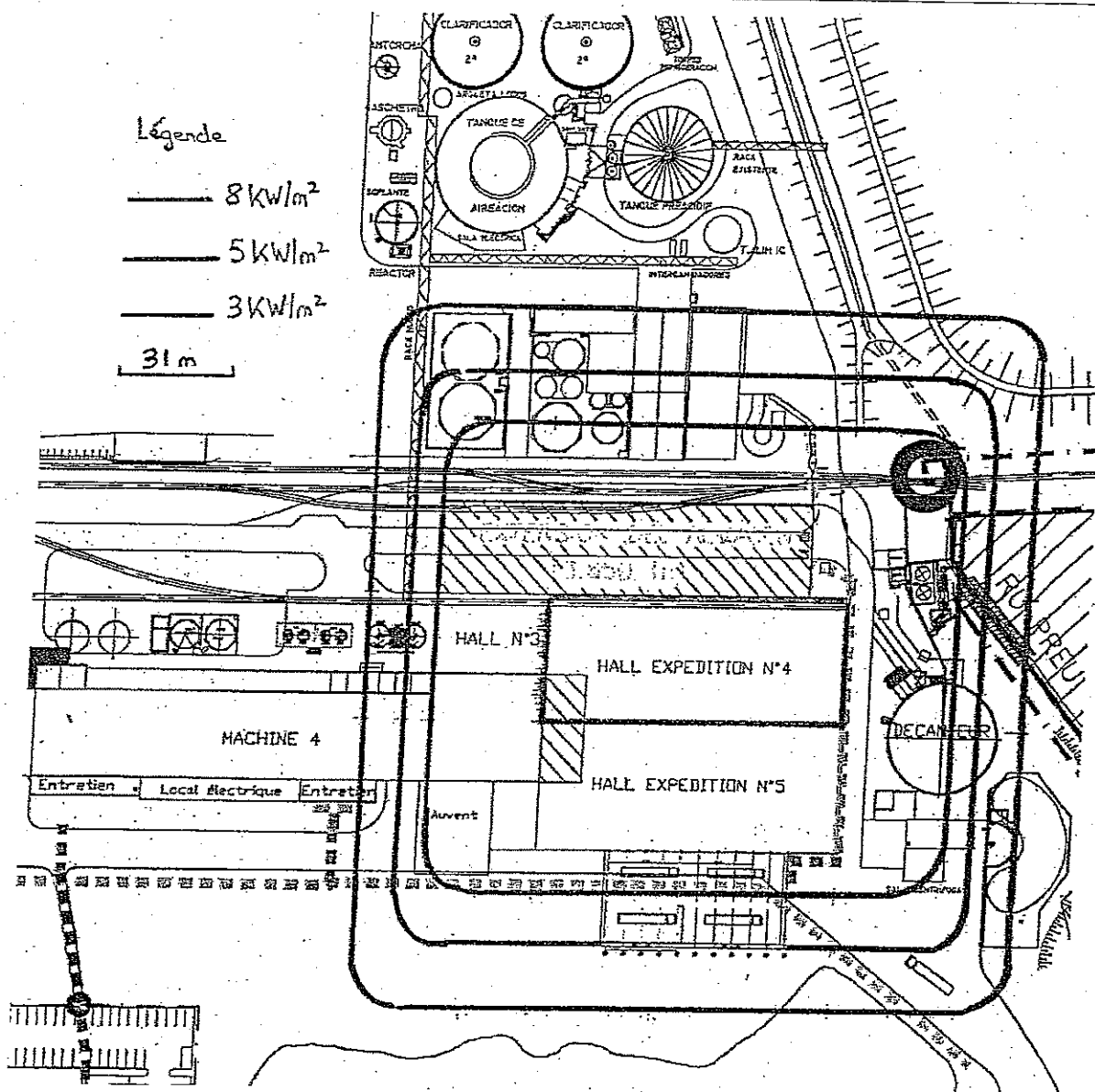
Fig. 74 : Distances d'effet pour l'incendie sur le hall 4
