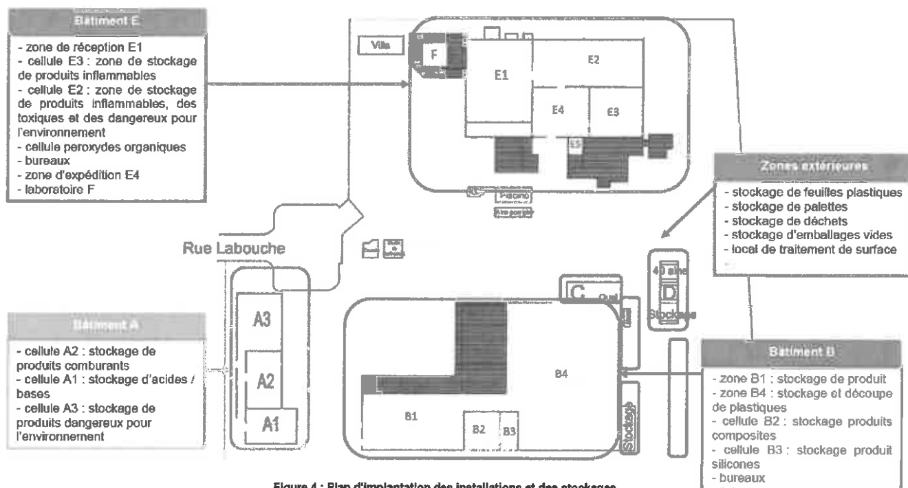
Figure 4 : Plan d'implantation des installations et des stockages
