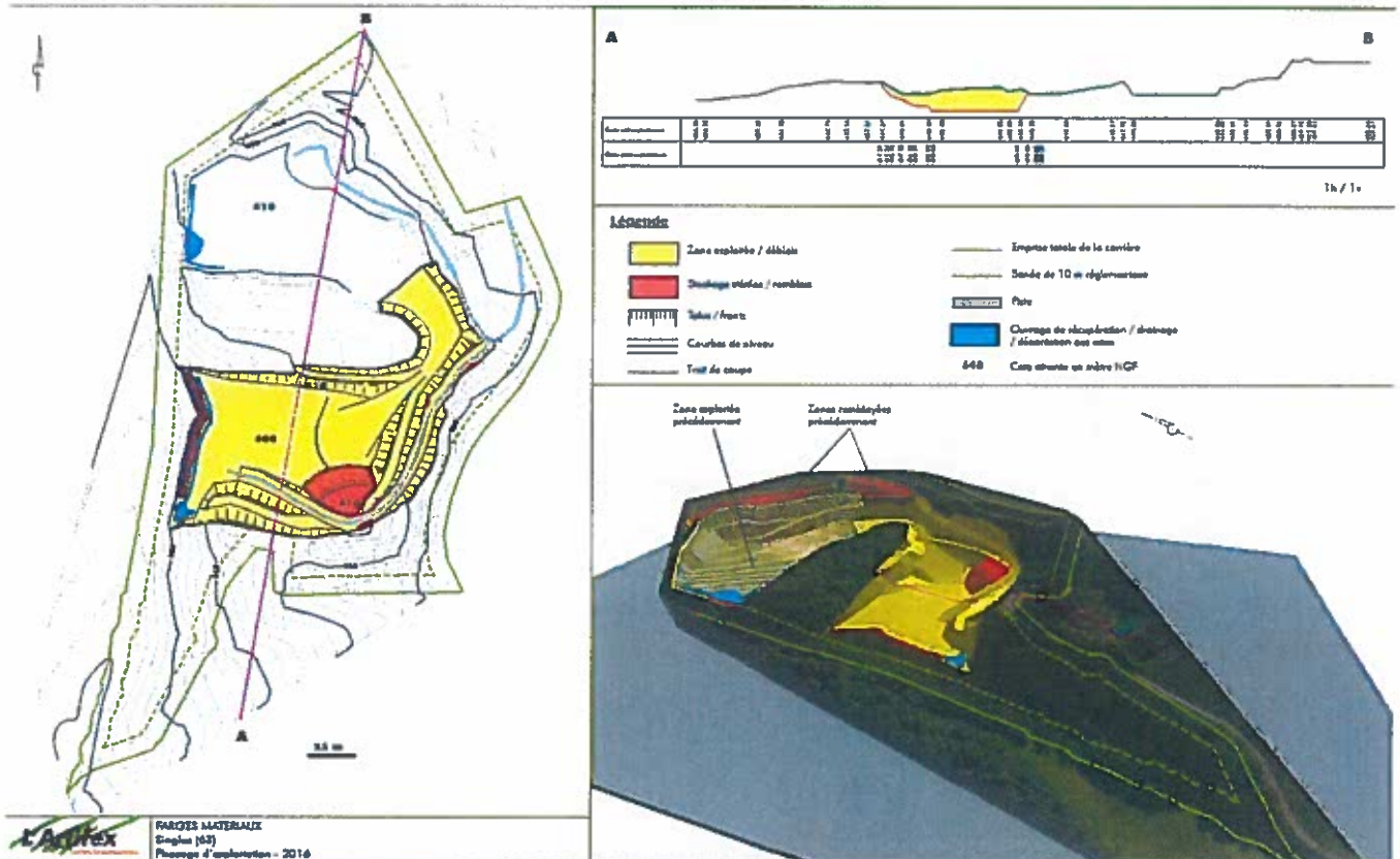
Figure 8 : Plan d'exploitation - Phase 2
