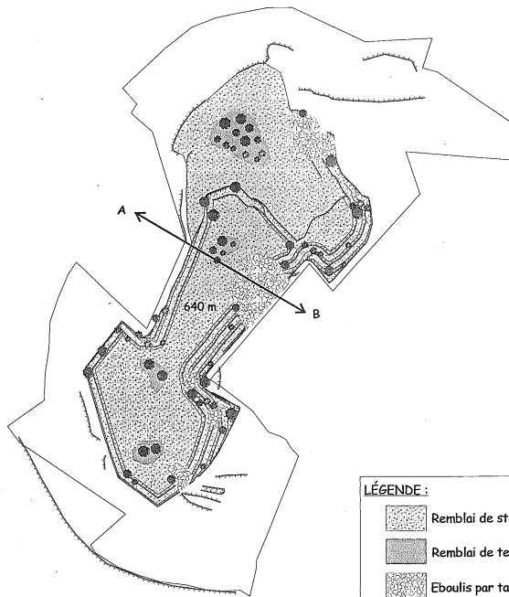
Figure 7 : Principe de remise en état du site
