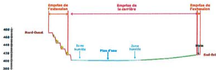
Coupe 2
