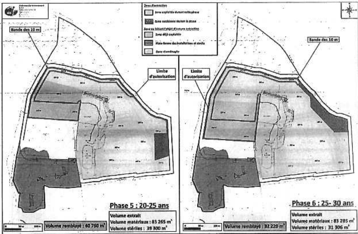
Figure 43 - Plans de phases d'exploitation au nord de la carrière - Phase 5 et Phase 6
