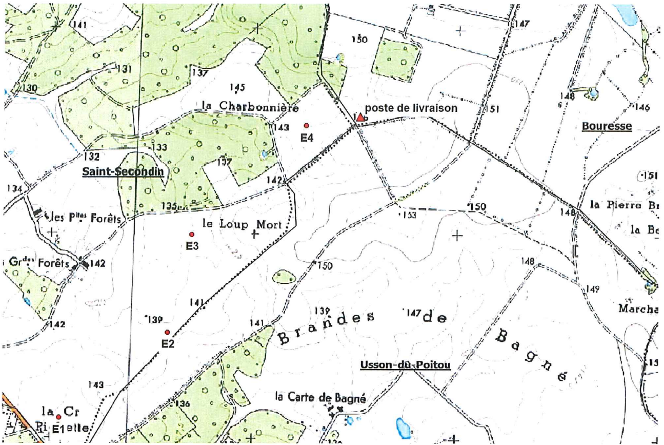
Plan de localisation des éoliennes et du poste de livraison
