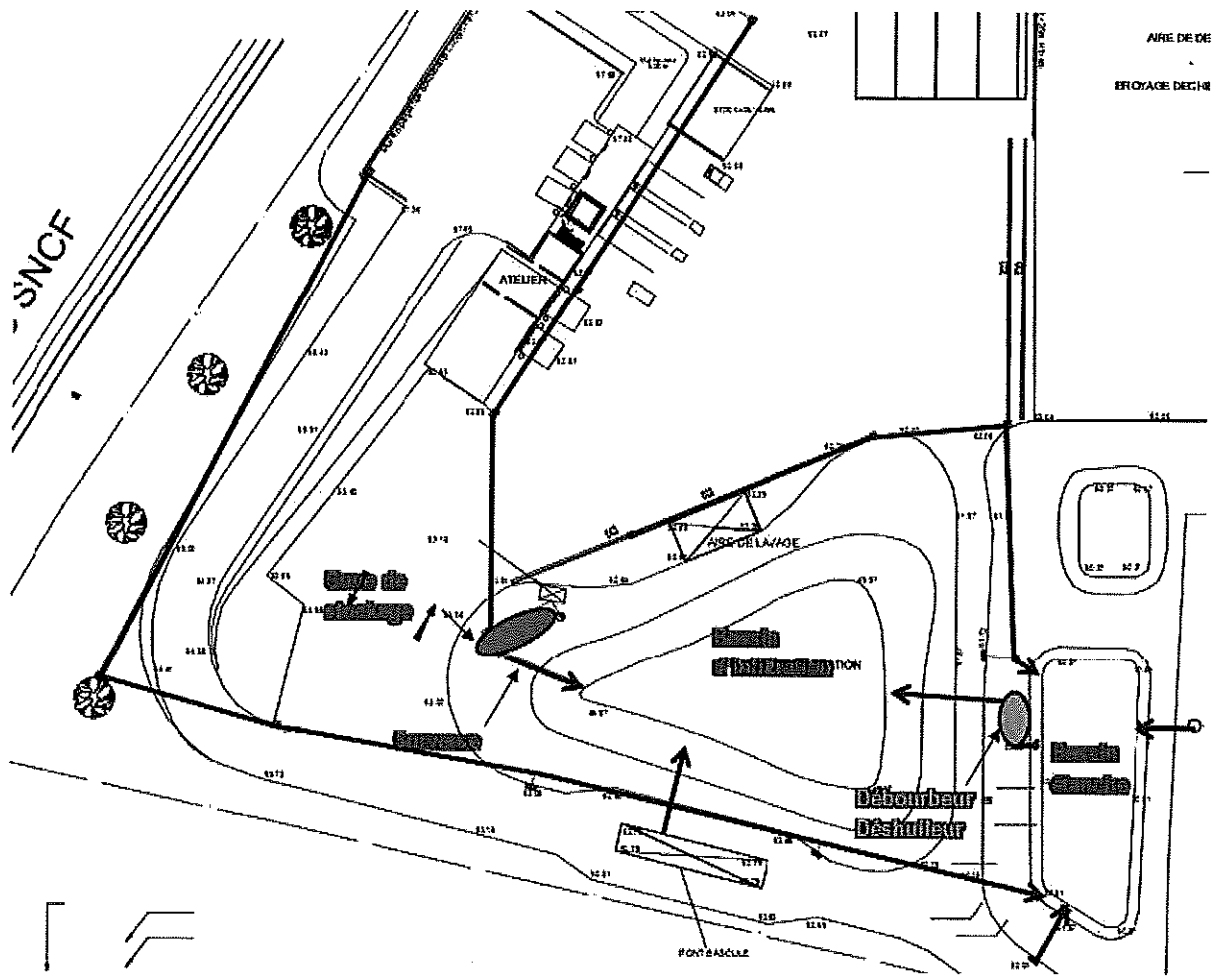
Figure 2 - Réseau de collecte des eaux pluviales actuel
