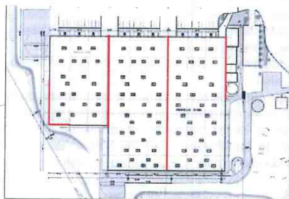
Localisation des murs REI 120 (en rouge) des cellules de stockage
