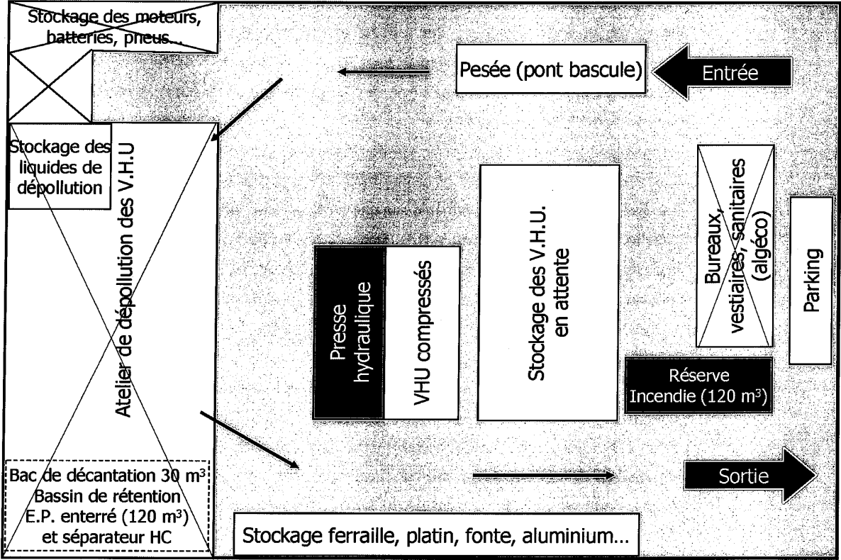
Synoptique de fonctionnement de l'installation
